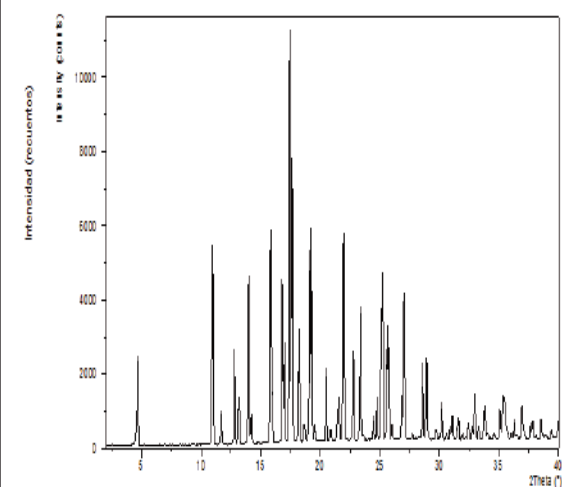
XRPD de L-lactato anhidrato 1 (AH1)
